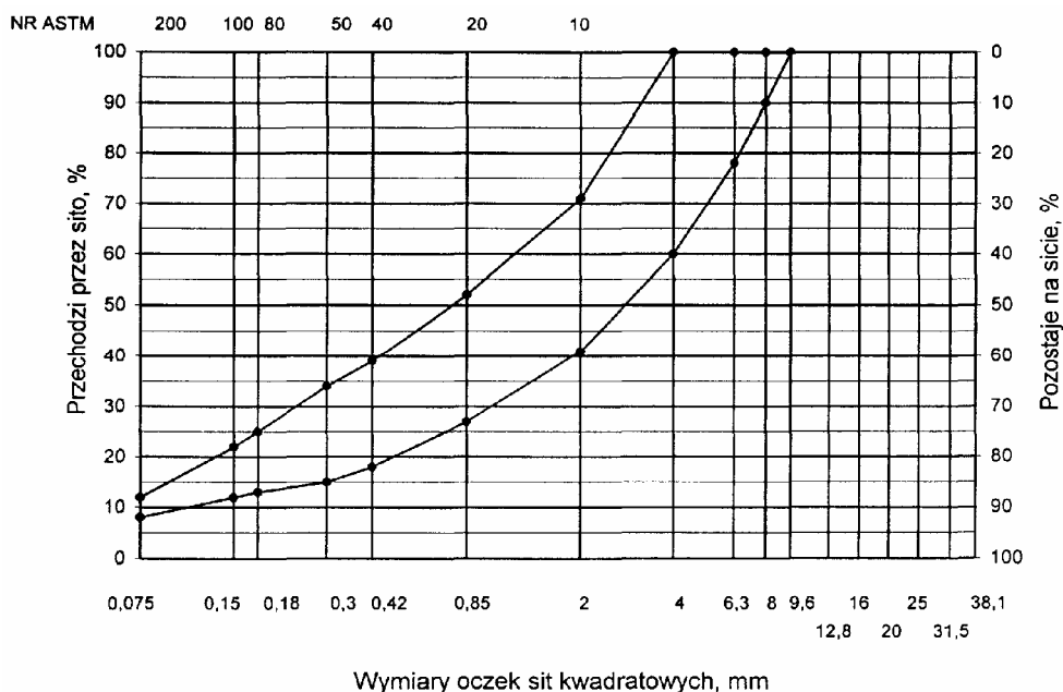
Rys. 3. Krzywe graniczne uziarnienia mieszanki mineralnej BA od 0 do 8mm, od 0 do 6,3 mm do warstwy ścieralnej nawierzchni drogi o obciążeniu ruchem nawierzchni drogi o obciążeniu ruchem KR1 i KR2
