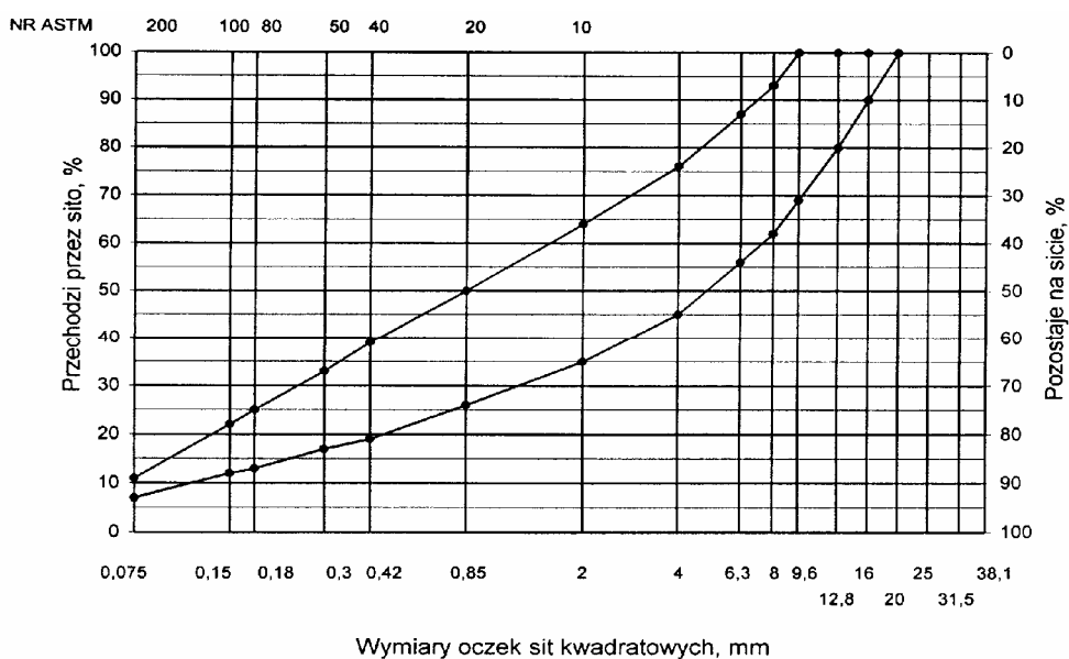
Rys. 2. Krzywe graniczne uziarnienia mieszanki mineralnej BA od 0 do 16mm, od 0 do 12,8 mm do warstwy ścieralnej nawierzchni drogi o obciążeniu ruchem KR1 i KR2
