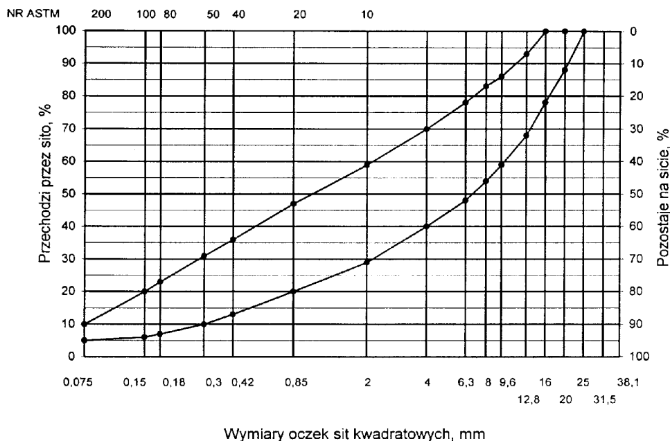
Rys. 1. Krzywe graniczne uziarnienia mieszanki mineralnej BA od 0 do 20 mm do warstwy ścieralnej nawierzchni drogi o obciążeniu ruchem dla KR1 i KR2
