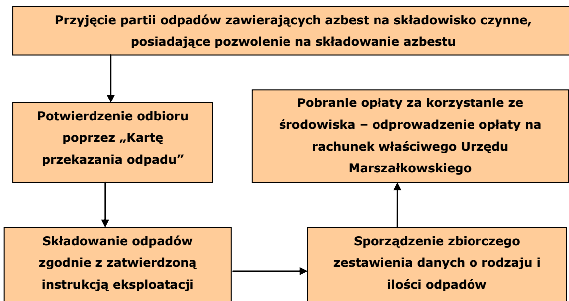
Rysunek 3. Schemat przekazania odpadów zawierających azbest do składowania.
